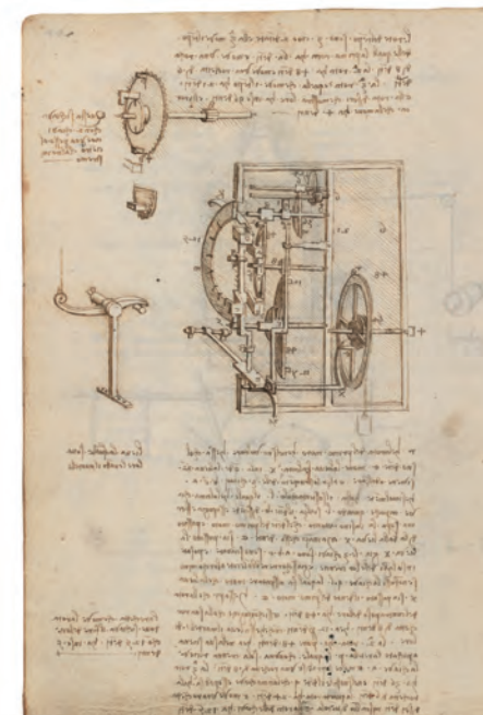
Mecanismo de un reloj. Codex Madrid I (Mss. 8937, f. 27v).
