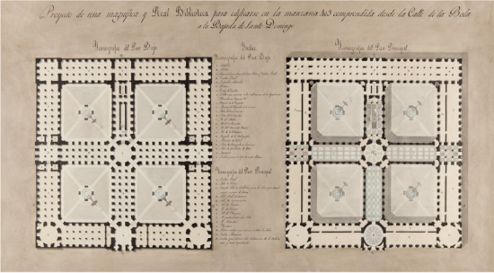
Plantas del proyecto de Aníbal Álvarez Bouquel para una Magnífica Biblioteca en la manzana 405 de Madrid. Primer premio de Primera Clase en 1831. Madrid, Real Academia de Bellas Artes de San Fernando. ASE A-777.
