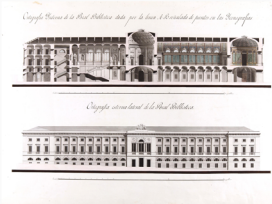
Sección longitudinal y alzado lateral del proyecto de Aníbal Álvarez Bouquel para una Magnífica Biblioteca en la manzana 405 de Madrid. Primer premio de Primera Clase en 1831. Madrid, ASE A-779.
